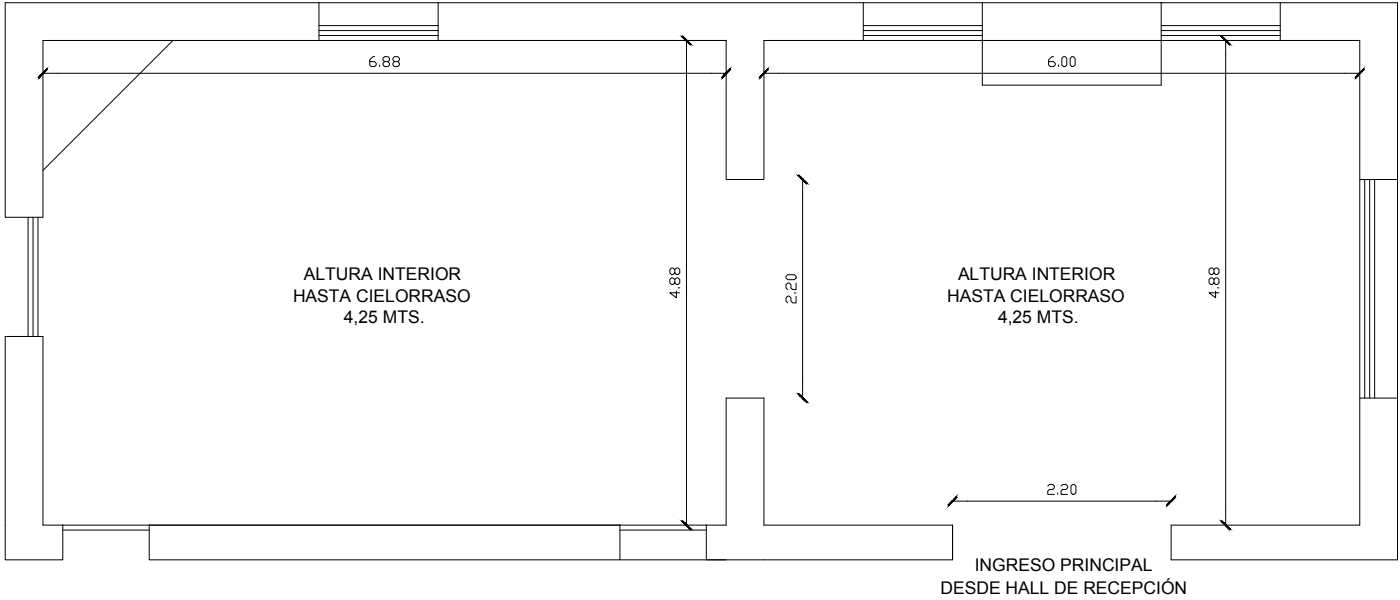
PLANTA BAJA
